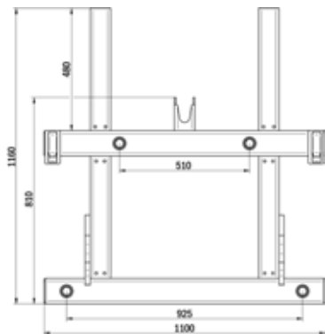
Uitvoering met verhoging met 4 rondebalentanden (2 tanden standaard)
