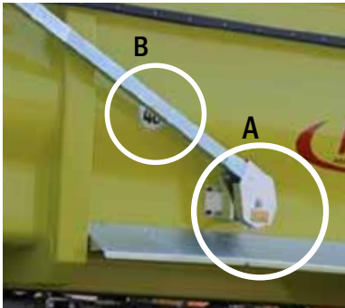
Hydraulische aandrijving via oliemotor – voor het oprollen van het net
