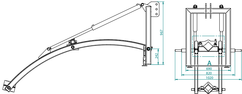
Hydraulisch opklapsysteem – kan worden gebruikt voor diepe putten
