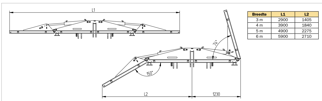
Ruimbreedte traploos instelbaar via de zijvleugels, opzetrooster (optioneel)
