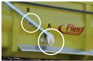
A) Optrekken door veerspanning B) Individuele lengteverstelling
