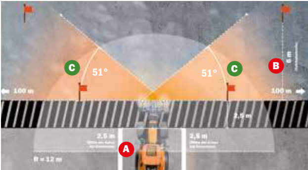
Het gecertificeerde camerasysteem voor kruisend verkeer
