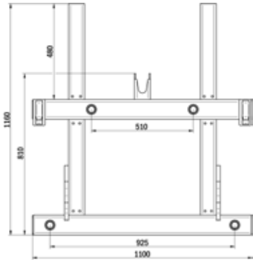
Uitvoering met verhoging met 4 rondebalemtanden (2 tanden standaard)
