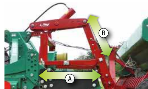
Horizontale (A) en verticale (B) trapeziumvormige delen
