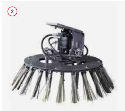
Staalkabelvechtwerk met kunststof mantel voor de beste onkruidverwijdering
