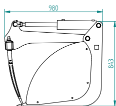
Conusbussen zijn al vastgelast in een robuuste tandendrager
