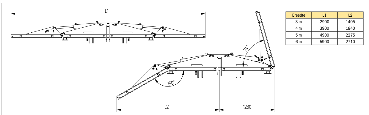
Ruimbreedte traploos instelbaar via de 2 zijvleugels, opzetrooster (optioneel)
