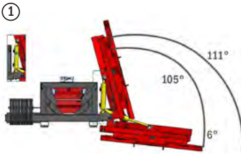
Kantelsysteem 111° - voor horizontaal en verticaal snoeien. De hoek kan daarbij traploos worden ingesteld.
