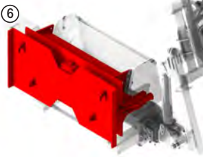
Overbelastingsbeveiliging als dempadapter: Bij een te hoge aanpersdruk kantelt de kop naar achteren ter bescherming tegen het blokkeren van de zaagbladen.
