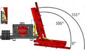
Kantelsysteem 111° - voor horizontaal en verticaal snoeien. De hoek kan daarbij traploos worden ingesteld.
