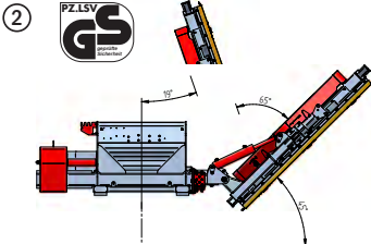
GS-certificering: Kantelsysteem 45° Het gekeurde type voldoet aan de eisen uit de Duitse productveiligheidswet (ProdSG) en de op dat moment geldende ervaringsgegevens inzake het voorkomen van ongevallen.
